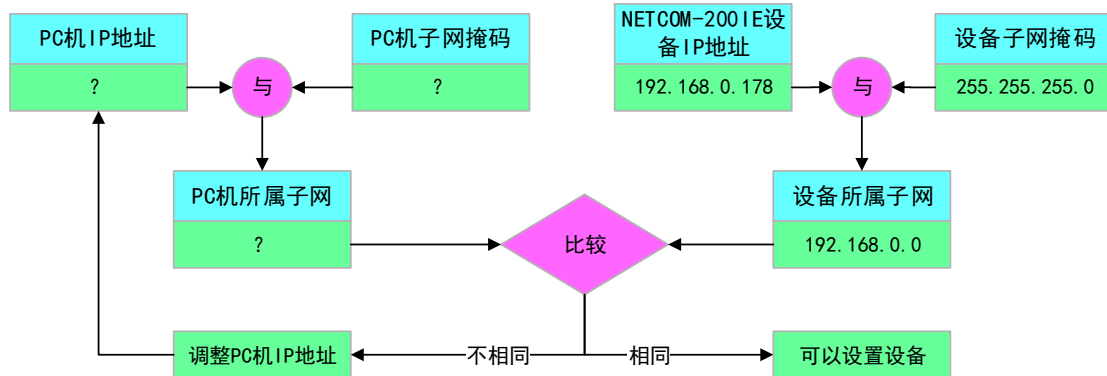
图 5.6 NETCOM-100IE+设备 IP 与 PC 机是否处于同一网段检查流程
