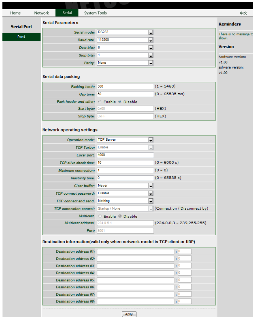
图 6.4 串口属性配置
