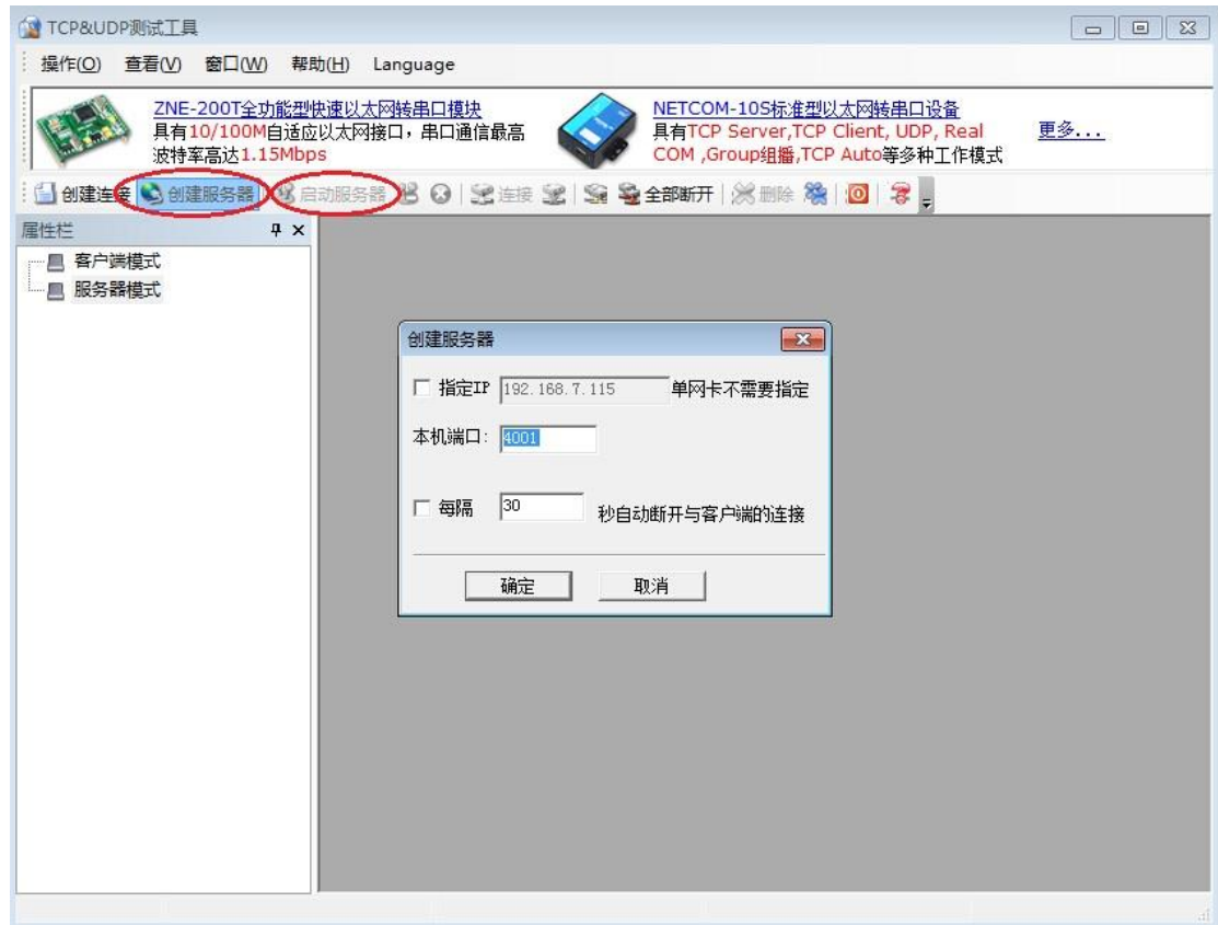
图 5.14 创建服务器
