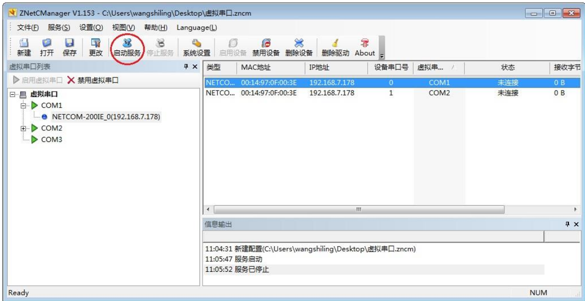
图 5.20 启动服务
