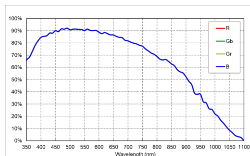
MV-CS020-60GM 量子效率
