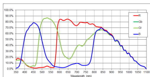
MV-CS020-60GC 量子效率
