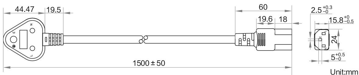
以色列_弯三插_C13_1.5 米:
