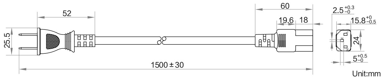
韩标_两插_C13_1.5 米:
