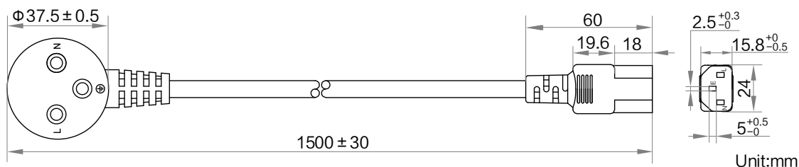
意标_三插_C13_1.5 米:
