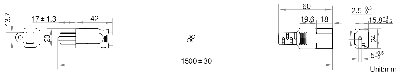
中国台湾_三插_C13_1.5 米:
