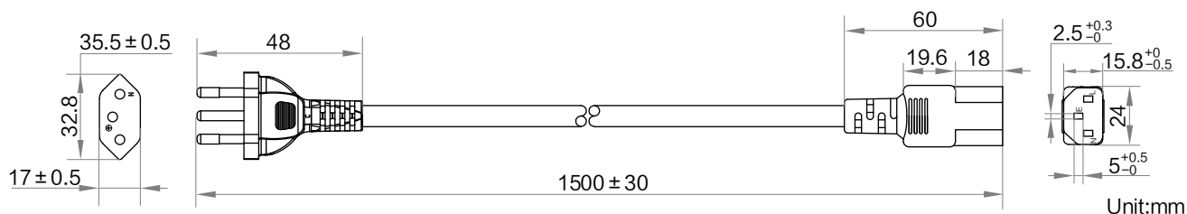
阿根廷_三插_C13_1.5 米:
