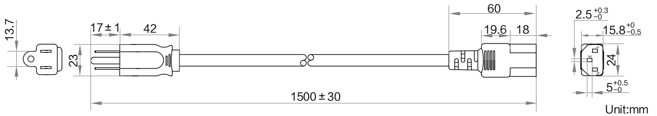
欧标_弯两插_C13_1.5 米:
