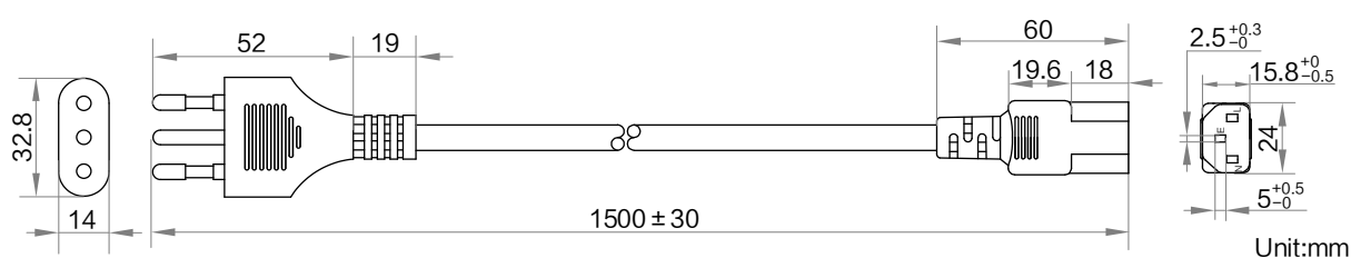
巴西_三插_C13_1.5 米:
