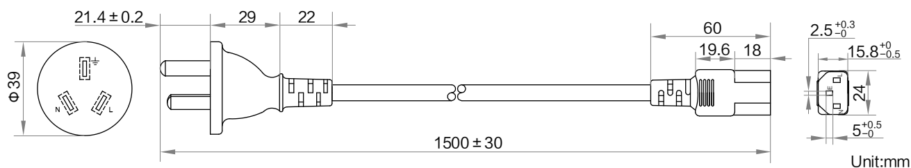
阿根廷_三插_C13_1.5 米:
