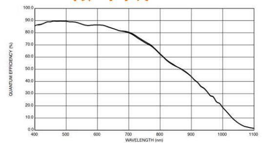
MV-CU200-20GM 响应曲线
