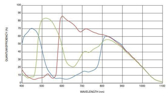
MV-CU200-20GC 响应曲线
