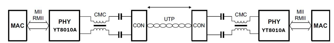
图 4.3 车载以太网典型网络连接示意图
