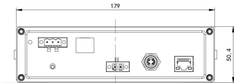
图 3.3 主机尺寸图三
