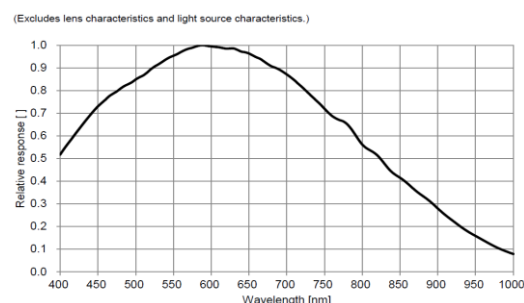
MV-CS020-10GM 量子效率
