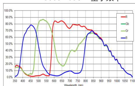
MV-CS032-60GC 量子效率
