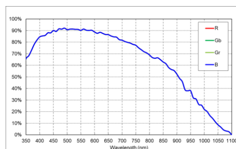
MV-CS032-60GM 量子效率
