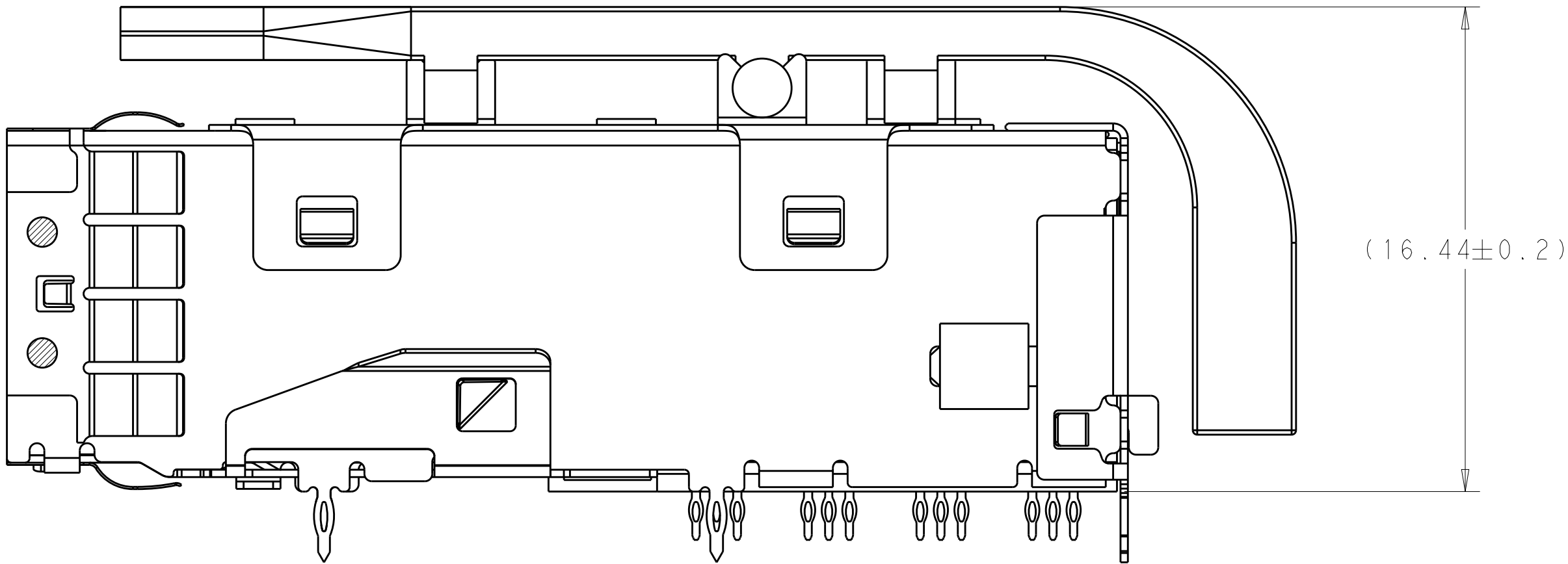
2198483-1 SCALE 6:1
