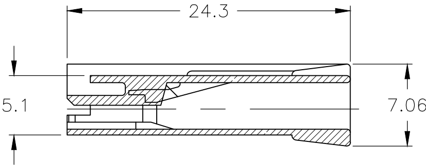
断面 A-A
